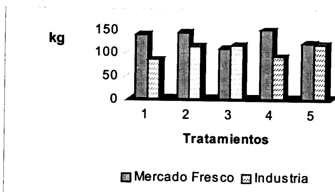
FIGURA 2: Kilogramos de fruta de mandarina Satsuma destinada a mercado fresco y a industria, promedios de las cuatro repeticiones en los dos años.
